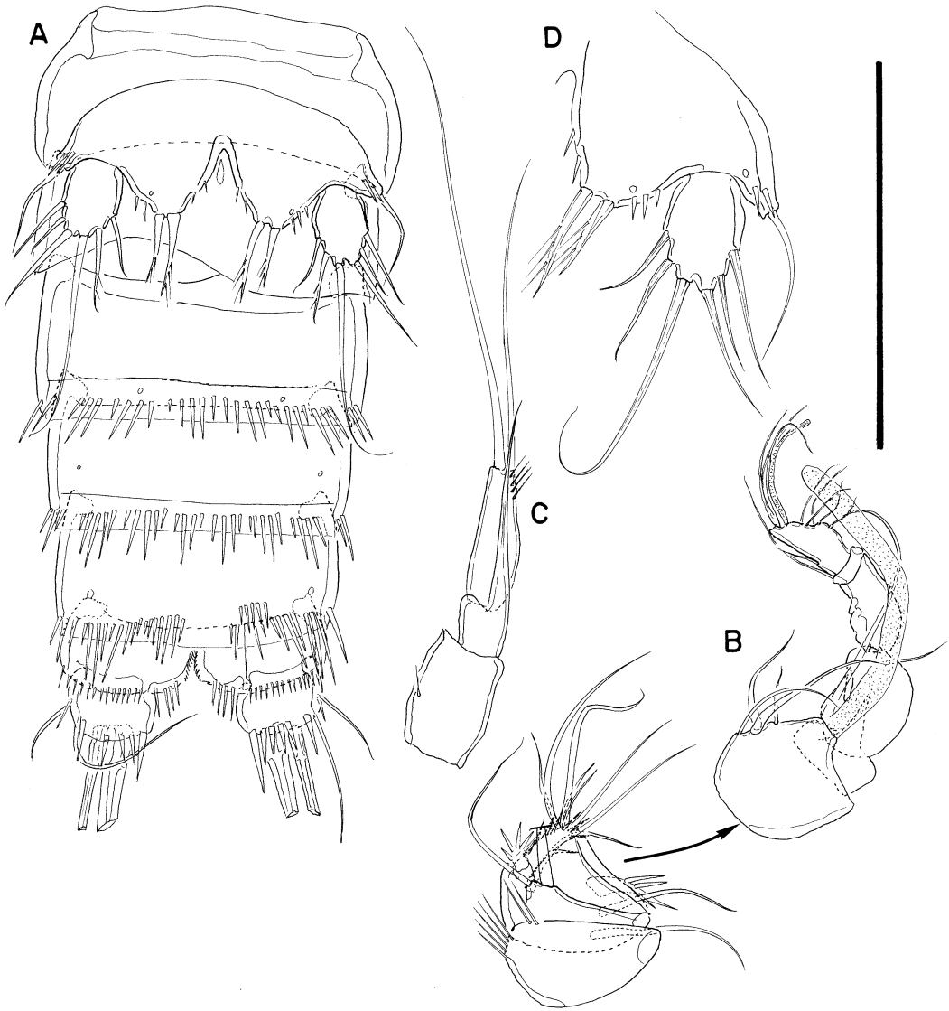
Figure 22. Mesochra freyri sp. nov., male. (A) Urosome, ventral; (B) antennule, ventral; (C) P3 ENP; (D) P5. Scale bar: 71 \mu m (A); 50 \mu m (B–D).
