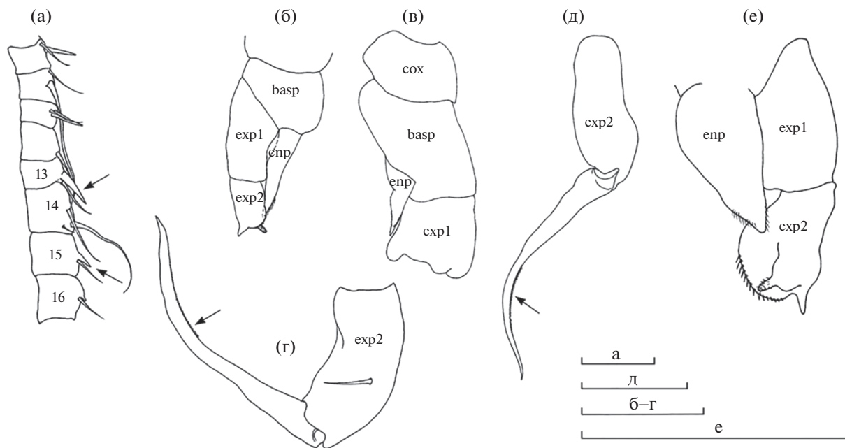
Рис. 2. Самец Leptodiptomus cf. angustilobus из р. Керженец (а–г) и из оз. Вера (д, е): а – средняя часть геникулирующей антеннулы (членики пронумерованы – 13, 14, 15, 16), б, е – левая P5; в – правая P5 (частично), г, д – экзоподит правой P5. Стрелками обозначены шипы и шипообразные выросты (а), а также хватательный коготь с шипиками (г, д). Остальные обозначения, как на рис. 1. Масштаб – 100 мкм.
