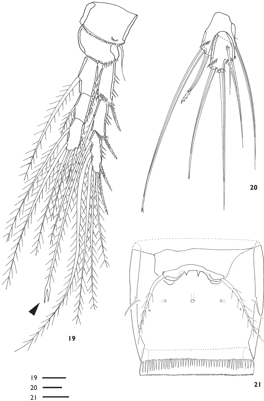
Figures 19-21. Chaulionyx paivacarvalhoi gen. et sp. n. ♀: 19 P4, anterior [seta with bifid apex arrowed] 20 P5, anterior 21 genital double-somite. Scale bars = 10 µm.
